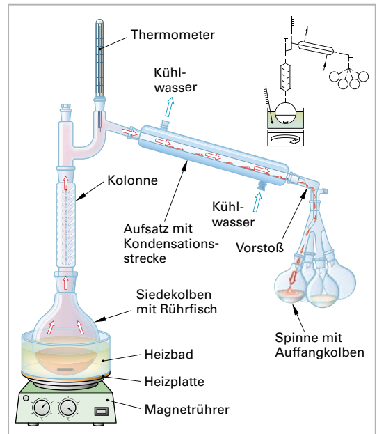
Bild 1: Aufbau einer Rektifikationsanlage
