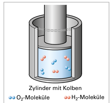
Bild 1: System und Umgebung
