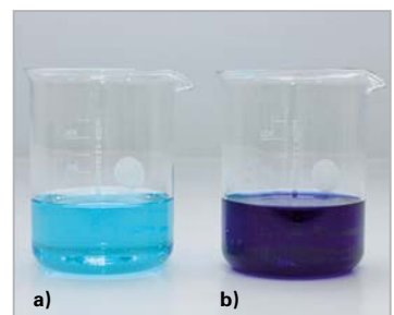
Bild 2: a) Kupfersulfat-Lösung, b) Tetraamminkupfer(II)-Lösung
