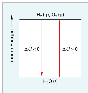
Bild 1: Innere Energie des Systems H_2/O_2 bzw. H_2O
